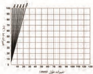
تغییرات طولی لوله های تک لایه پلی پروپیلن
